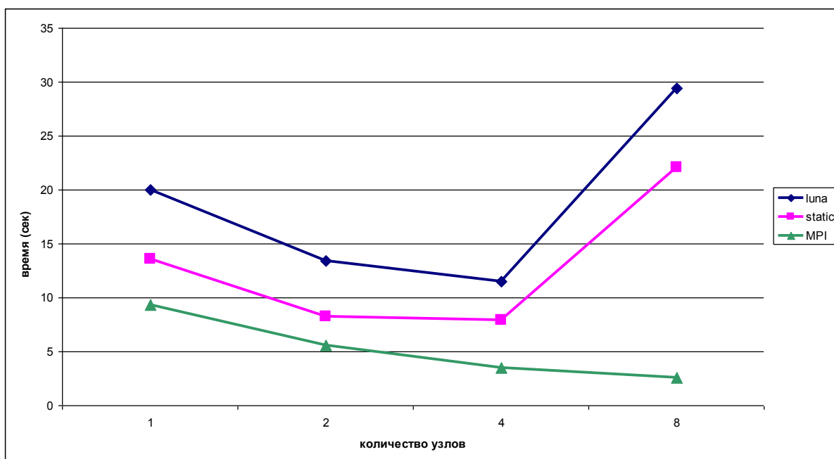
Рис. 7 Время исполнения ФП параллельного алгоритма редуцирования данных в зависимости от количества узлов (размер ФД 40x40x40, количество ФВ 10000, размер группы 250, количество редуций 10, количество потоков 4)
