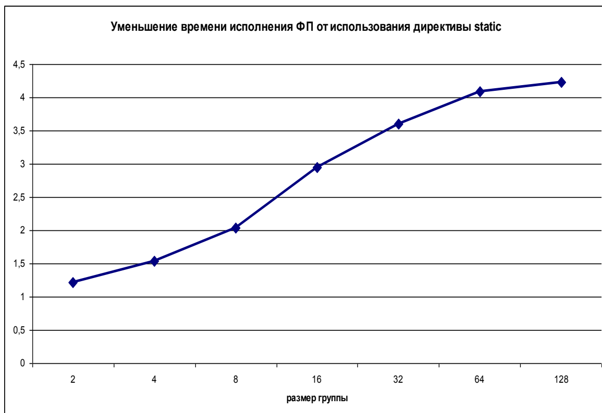
Рис. 3 Уменьшение времени исполнения ФП от использования директивы static в зависимости от размера группы (размер ФД 10x10x10, количество редукций 200)
