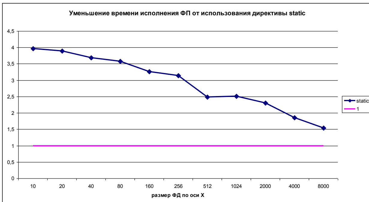
Рис. 6 Уменьшение времени исполнения ФП от использования директивы static в зависимости от размера ФД по оси X (количество редукции 200, размер группы 64, размер ФД по оси Y и Z 10)
