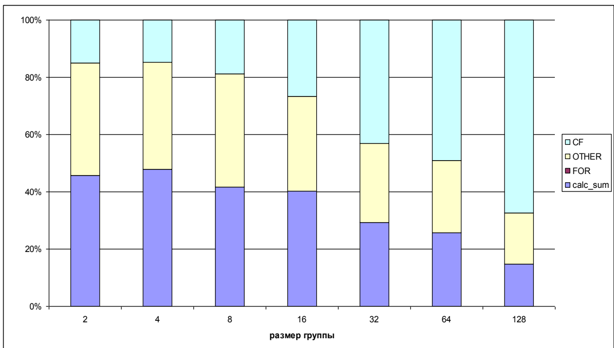
Рис. 5 Процентное соотношение времени исполнения ФП с использованием директивы static в зависимости от размера группы
