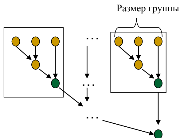
Рис. 2 Схема информационных зависимостей между ФВ во ФП для параллельного алгоритма редуцирования данных.
