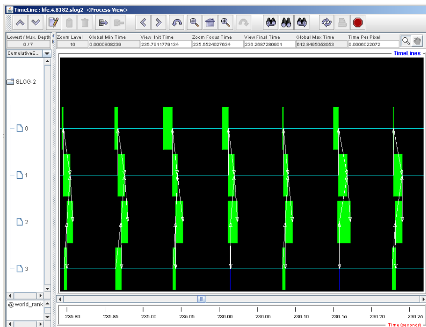
Рис. 5. Просмотр с большой детализацией для малых промежутков времени в окне
