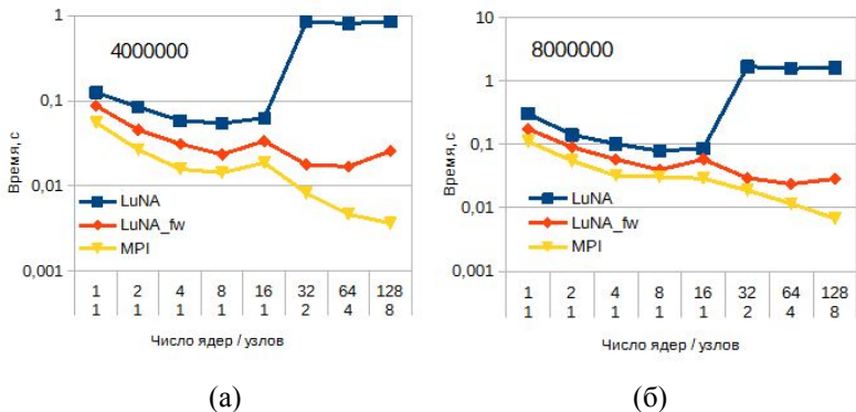
Рис. 4. Сравнение производительности различных реализаций алгоритма IADE-RB-CG: размер задачи 4000000 узлов (а) и 8000000 узлов (б)
