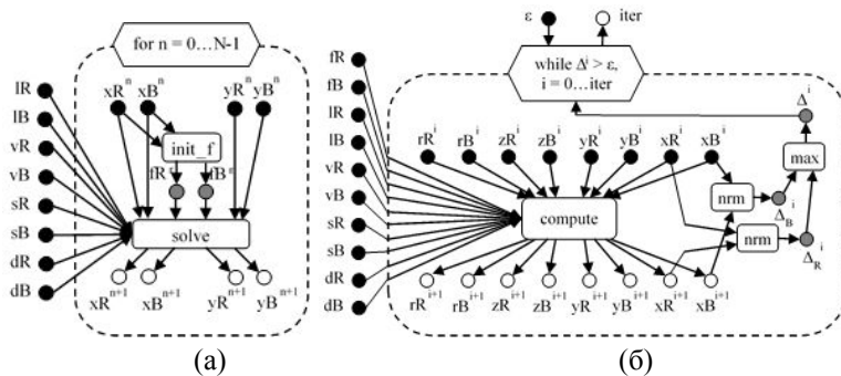
Рис. 1. Фрагментированный алгоритм метода IADE-RB-CG (a) и фрагментированный алгоритм, реализующий фрагмент кода "solve" (б)
