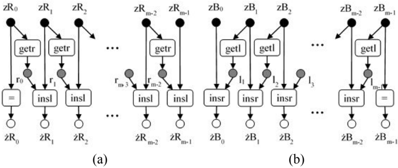
Рис. 3. Фрагментированные алгоритмы передачи границ подобластей: правой (а) и левой (б)
