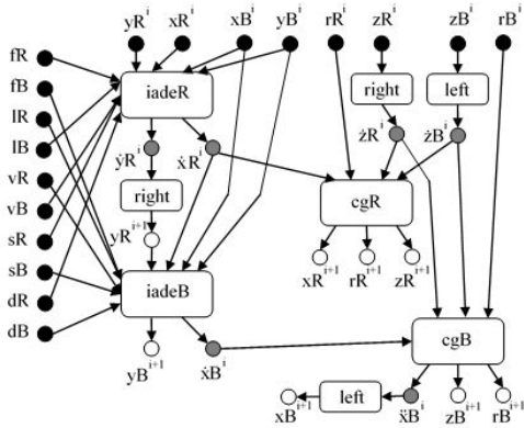
Рис. 2. Фрагментированный алгоритм i -й итерации метода IADE-RB-CG
